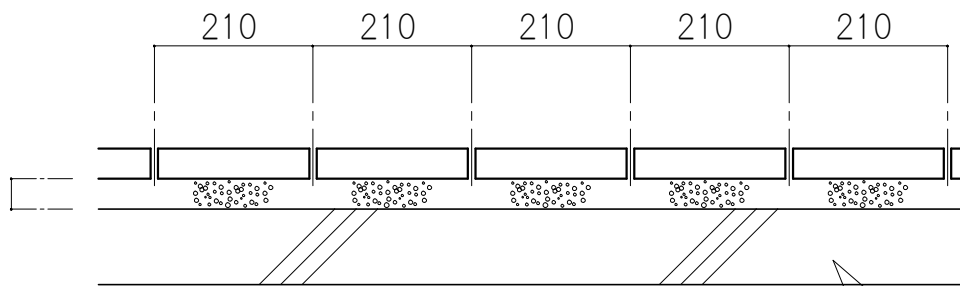
重ね瓦割り図
