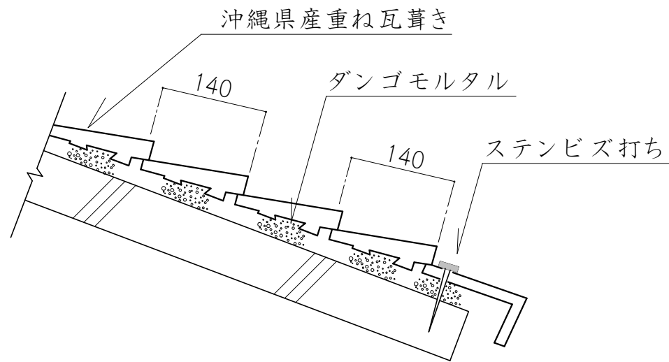
断面施工図
