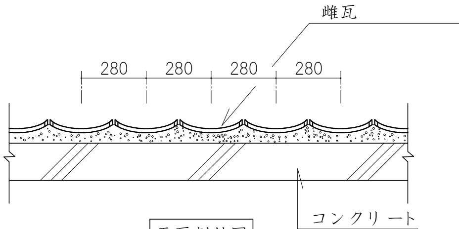
平瓦割付図
